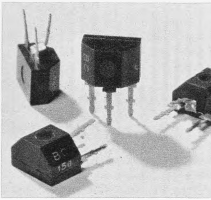
Bild 3c. Fertige Einzeltransistoren in Plastikgehäusen vom Typ BC 158
