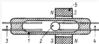
Bild 7. Kugelanker-Kontakt.
