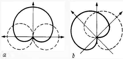
Bild 2. Richtcharakteristiken von Stereo-Doppelmikrofonen; a = MS-Aufstellung, b = XY-Aufstellung
