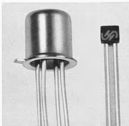
Bild 1. Größenvergleich zwischen dem Metalltransistorgehäuse TO-18 und einem Subminiatur-Kunststoffgehäuse (Werkaufnahmen: Siemens)
