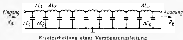
Ersatzschaltung einer Verzögerungsleitung
