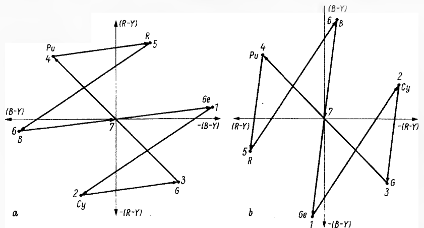
Bild 103. a = Zeigerdiagramm bei Verwendung eines Oszillografen mit ungeradzahligen Verstärkerstufen im X-Kanal, b = Zeigerdiagramm, wenn dem X-Verstärkereingang das (R - Y)-FD-Signal, dem Y-Eingang das (B - Y)-FD-Signal zugeführt wird
