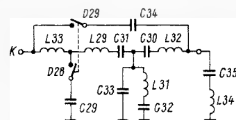
Bild 2. Prinzipschaltbild des VHF-Eingangskreises
