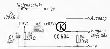
Bild 2. Torschaltung mit einem Nf-Transistor
