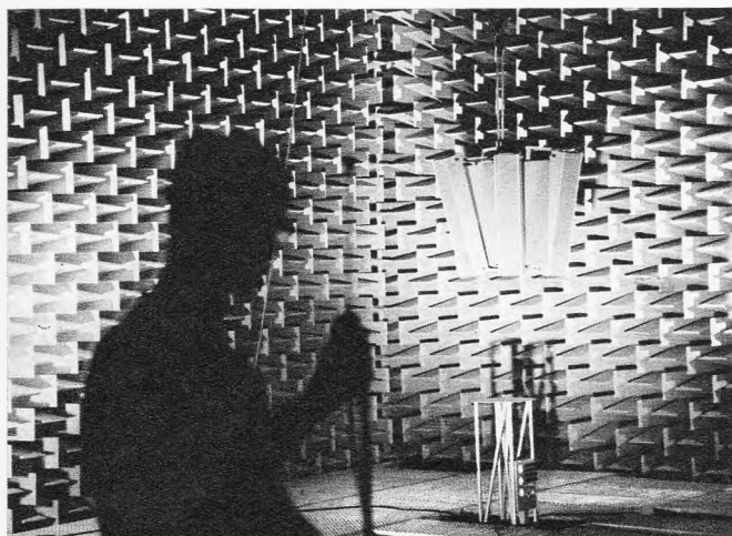
Links: Bild 1. Das Innere des schalltoten Raumes im Labor für technische Akustik der Siemens-Werke in Karlsruhe
