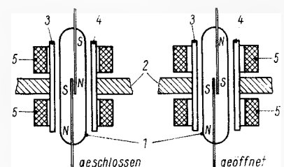
Bild 8. Ferreed-Relais.
