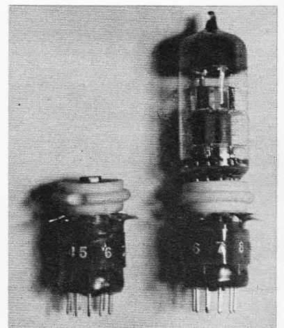
Rechts: Bild 3.09-1. Adaptersockel zum Spannungsmessen an unzugänglichen Röhrenfassungen
