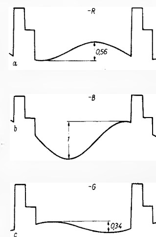
Bild 100. Farbauszugssignale einer Regenbogenfarbfolge an den Katoden der Farbbildröhre bei RGB-Ansteuerung
