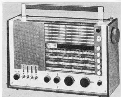
Reiseempfänger, Modell Supernova, mit zehn Empfangsbereichen, KW-Lupe mit Kapazitätsdiode, mit vorabstimmbareren Tasten für vier UKW-Programme und eingebautem Netzteil mit automatischer Batterie/Netzumschaltung (Aufnahme: Blaupunkt)
