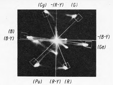
Bild 102. Zeigerdiagramm, wenn bei RGB-Ansteuerung den Eingängen des X-Y-Oszillografen die negativen Farbdifferenzsignale - (R - Y) und - (B - Y) zugeführt werden
