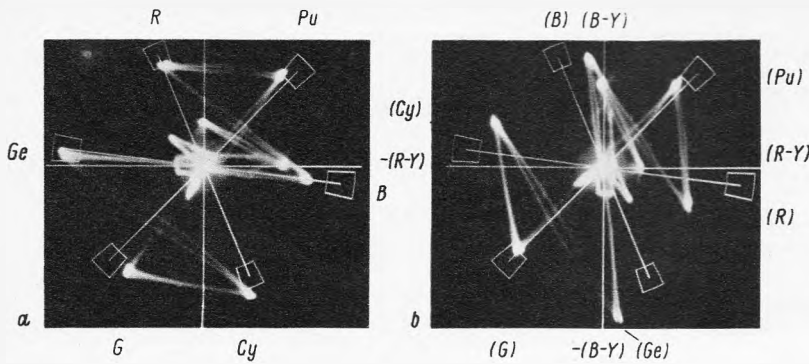
Bild 101. a = Zeigerdiagramm einer Farbbalkenfolge (Treppnbalken), b = Zeigerdiagramm, wenn dem X-Y-Oszillografen nicht das (R - Y)- und das (B - Y)-FD-Signal, sondern das - (R - Y)- und das - (B - Y)-FD-Signal zugeführt werden
