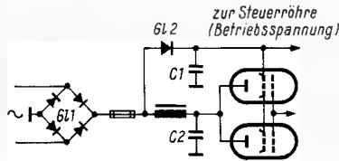
Die vorgeschlagene stromsparende Schaltung für ein Netzteil
