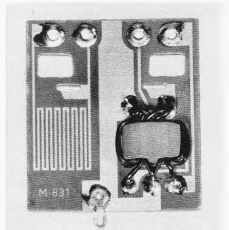
Bild 4. Antennenüberträgerplatte zum Kanalwähler, bestehend aus einer Hartpapierplatte mit gedruckter Verdrahtung. Für VHF wird ein Guanella-Überträger, bei UHF eine gedruckte \lambda/2 -Umwegleitung verwendet
