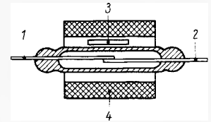
Bild 4. Schutzgaskontakt-Relais mit Ruhekontakt (Öffner). 1, 2 = Kontaktzungen, 3 = Dauermagnet, 4 = Erregerspule
