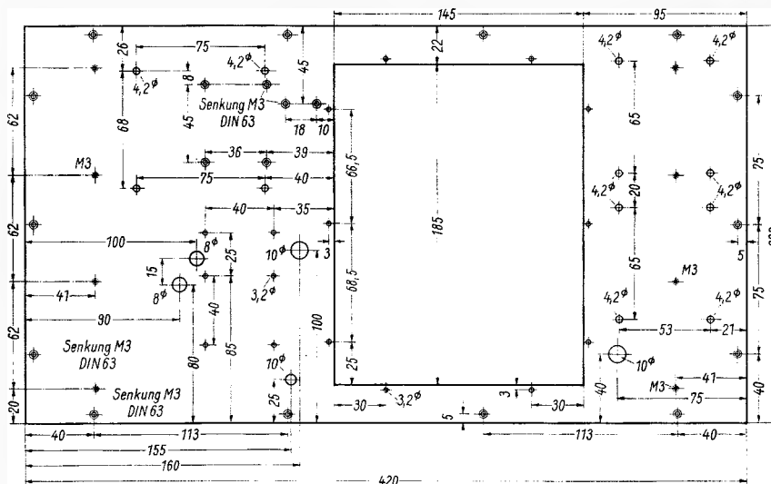
Bild 4. Größe und Maße des Chassisbodens
