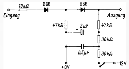
Bild 1. Torschaltung mit zwei Siliziumdioden
