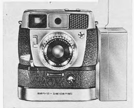
Baldamatic-Kleinbildkamera mit Automatik-Untersatz und angebautem Empfänger der Metatron-Funkfernsteuer-einrichtung
